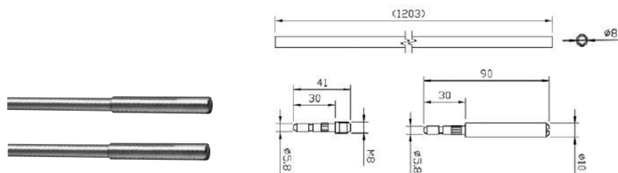
Kit aste per anta secondaria
