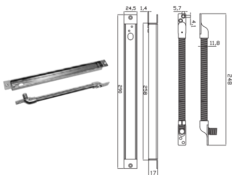
Passacavo flessibile da incasso L = mm 260 Apertura fino a 90°
