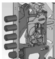
J Sistema di autobloccaggio del catenaccio (Self Locking System)
