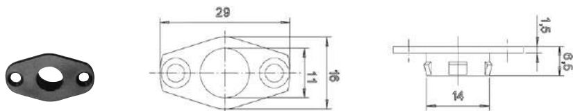
Guida aste inferiore per anta secondaria
