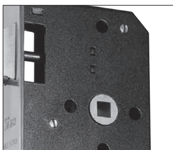
Cassa chiusa e fori passanti
