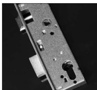
Cassa chiusa e fori passanti
