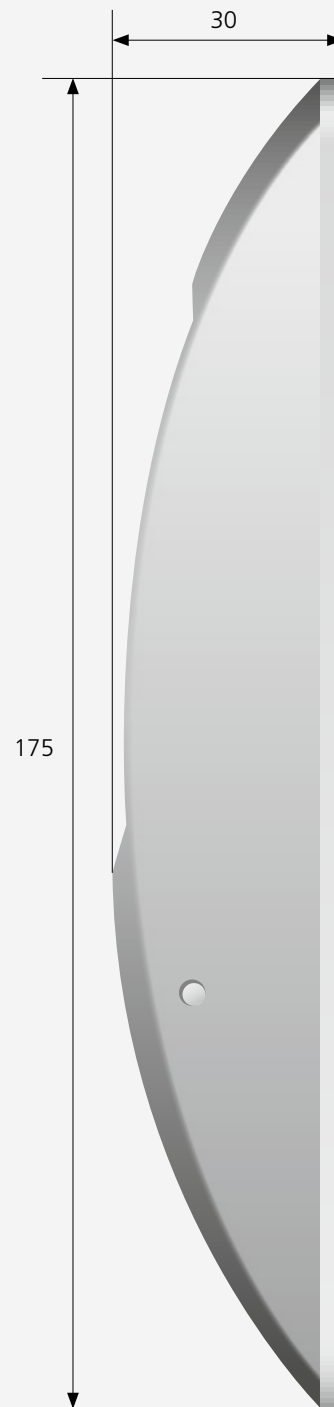
Seitenansicht
