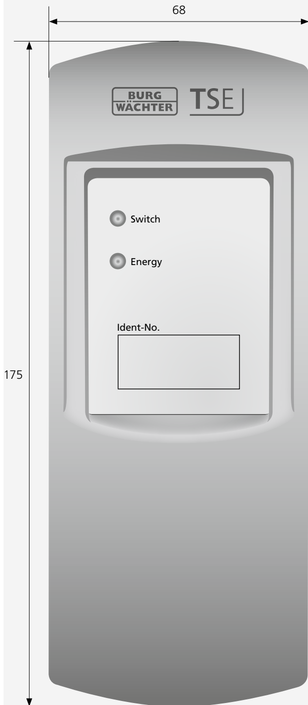
Frontansicht
